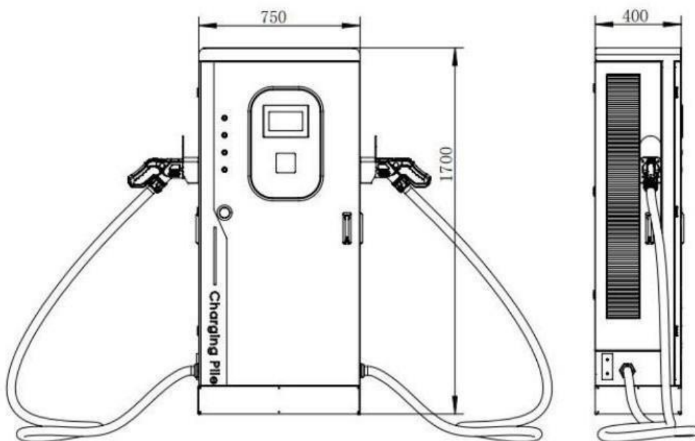
Obrázek 5-1-2 Rozměry zařízení (Ares DC-60kW/80kW)
