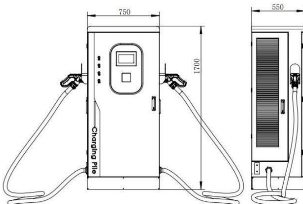
Obrázek 5-1-3 Rozměry zařízení (Ares DC-120kW/160kW)
