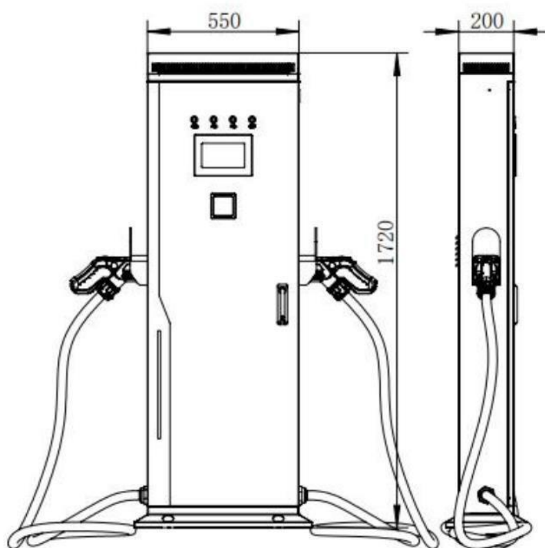
Obrázek 5-1-1 Rozměry zařízení (Ares DC-30kW/40kW)
