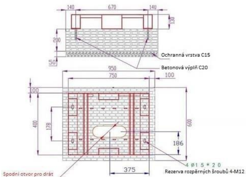
Schéma způsobu instalace 60Kw-80Kw DC nabíjecí stanice
